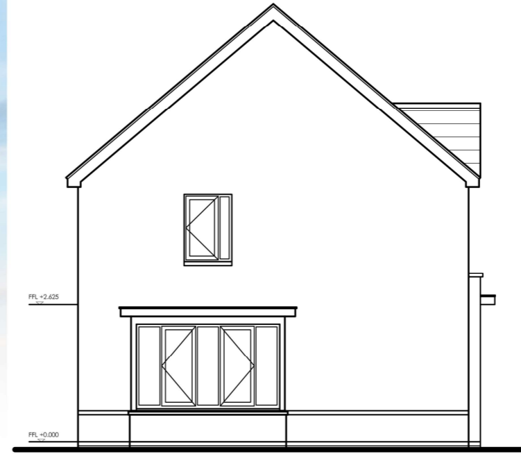
Side/Front Elevation
