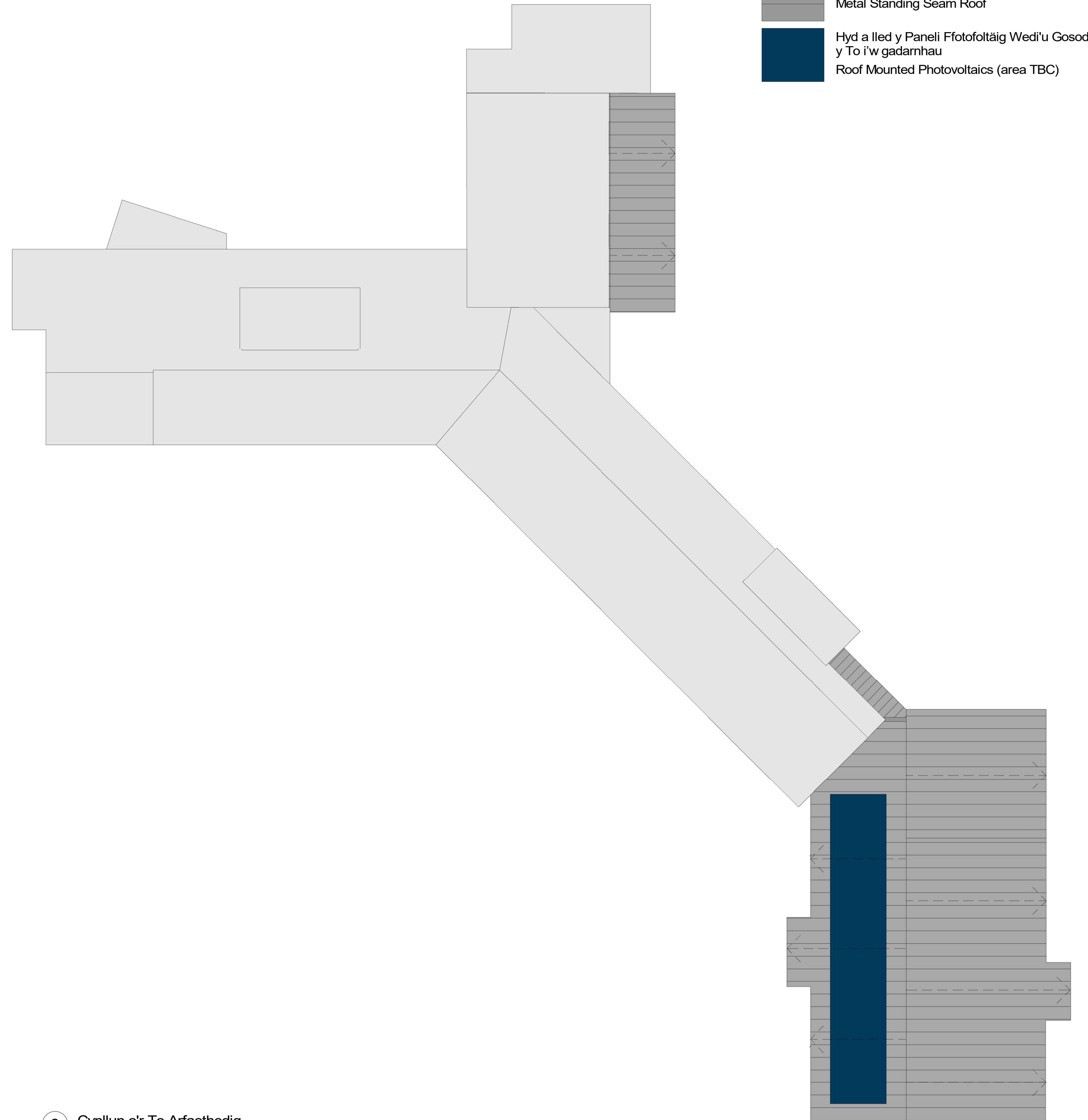
2 Cynllun o'r To Arfaethedig Proposed Roof Plan 1:200
